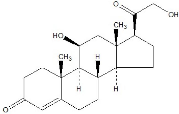
Corticosterone
